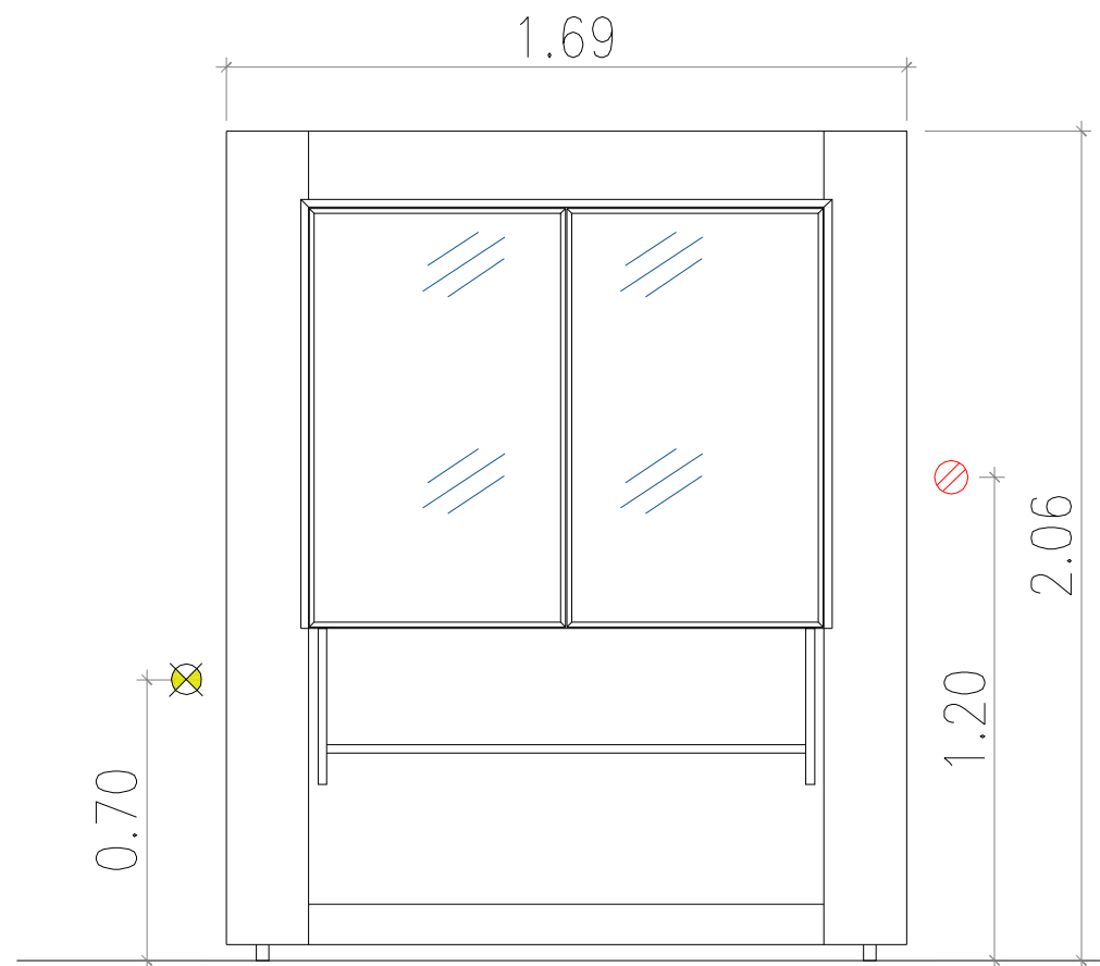
ELEVACIÓN
