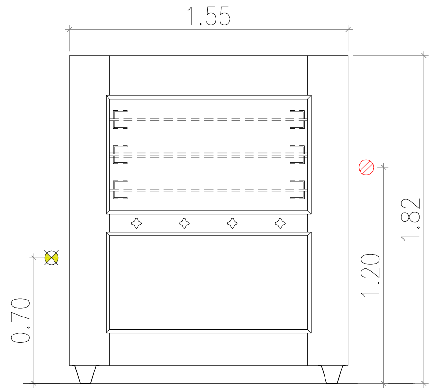
ELEVACIÓN
