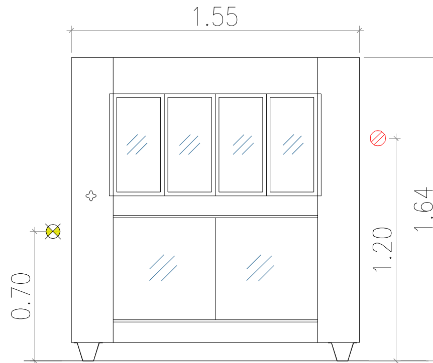
ELEVACIÓN
